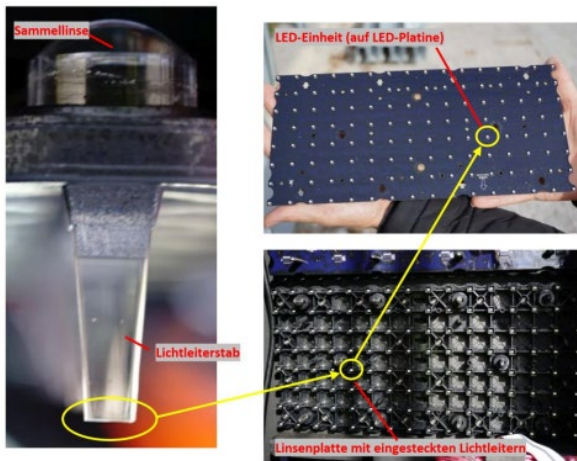
Abbildung 4: Sammellinse mit Lichtleiterstab, Trägerplatte und LED-Platine
