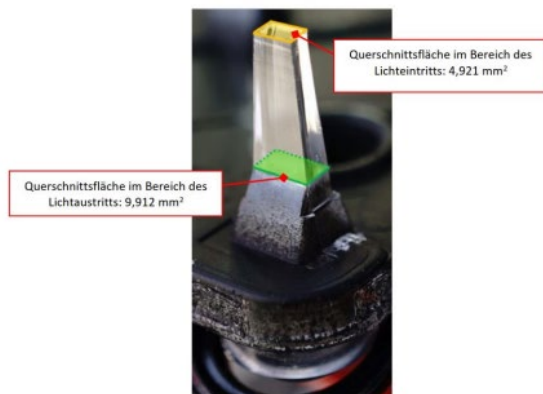
Abbildung 7: Verdeutlichung der allmählichen Zunahme des Querschnitts des Lichtleiterstabes
