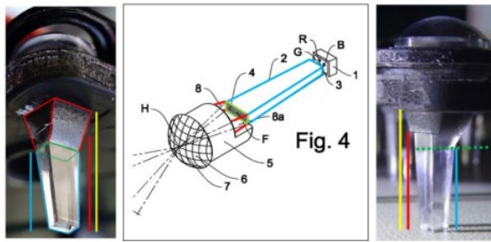
Abbildung 6: Gegenüberstellung des Eingriffsgegenstandes gemäß Gutachten K 12 (links) des IOSB-Messberichts Beilage 5 13 (rechts) und der in Fig. 4 des Streitpatents dargestellten Ausführungsform der Erfindung (mitte) mit jeweils hinzugefügter Markierung des Lichtleiterstabes (blau), der Lichtaustrittsfläche (grün) und weiterer optischer Geometrie im Bereich der Sammellinse gemäß Absatz [0054] des Streitpatents
