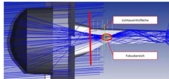
Abbildung 8: Verlauf der Lichtaustrittsfläche durch den Fokusbereich der Sammellinse gemäß Abbildung 18 (untere Darstellung) des IOSB-Messberichts Beilage 5 13
