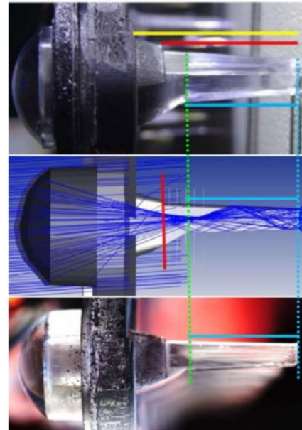
Abbildung 5: Wiedergaben von Abbildungen der eingriffsgegenständliche Optik aus dem IOSB-Messbericht Beilage 5 13 und dem Gutachten K 12, jeweils mit Markierung des Lichtleiterstabes (blau) und der Lage der Lichtaustrittsfläche (grün)
